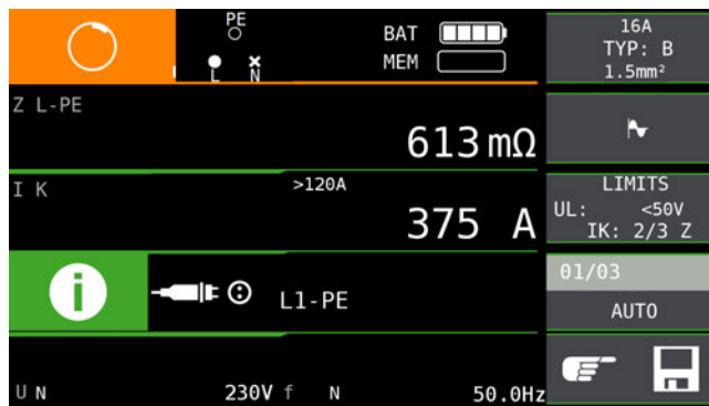
Anzeige Schleifenwiderstandsmessung
